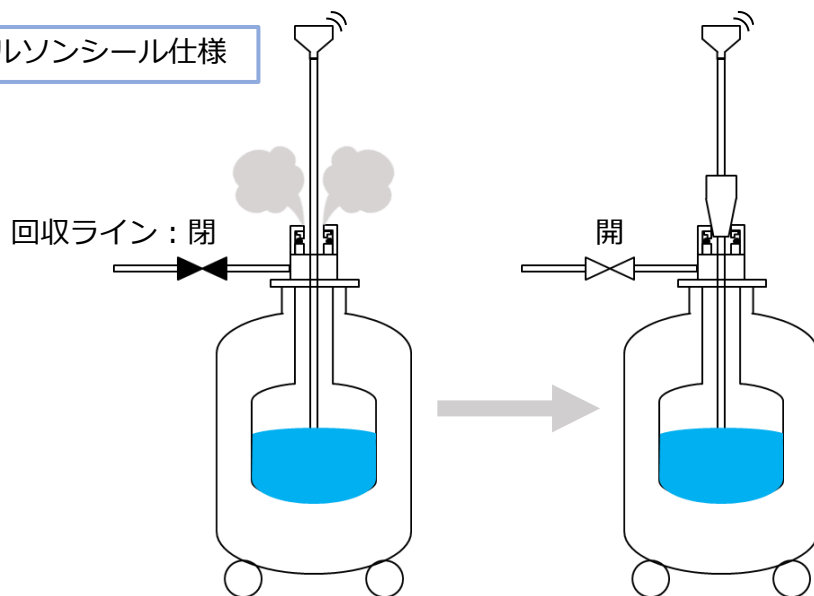
ダイナミックシール仕様
